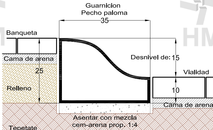
CORTE INSTALACION DE GUARNICION EN CAMELLONES Delimitando áreas verdes
