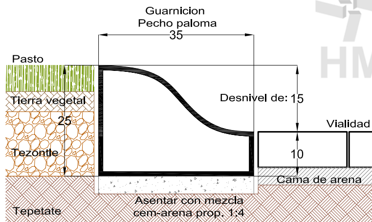
CORTE INSTALACION DE GUARNICION EN BANQUETA Delimitando áreas peatonales
