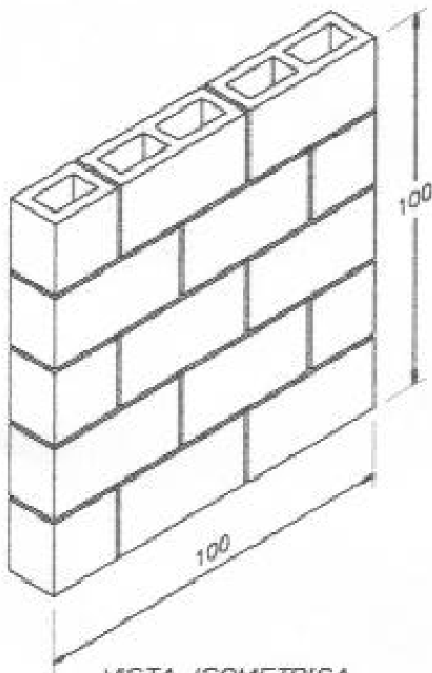
VISTA ISOMETRICA
